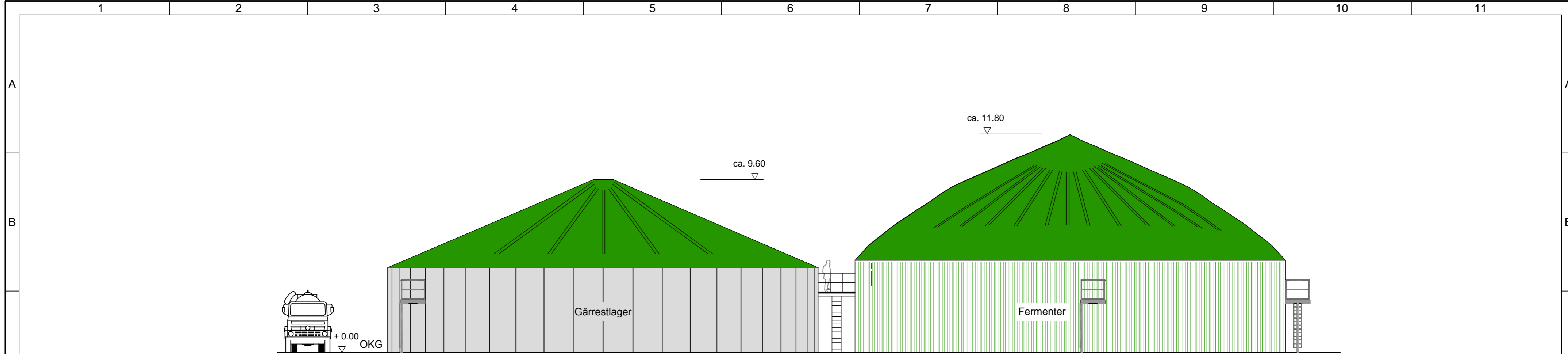
Nordansicht
